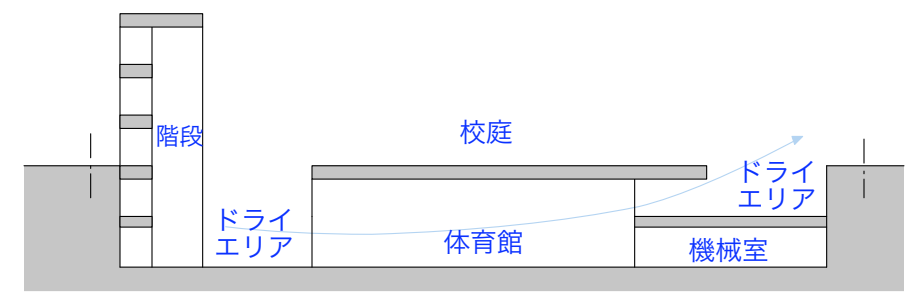
東西断面図
