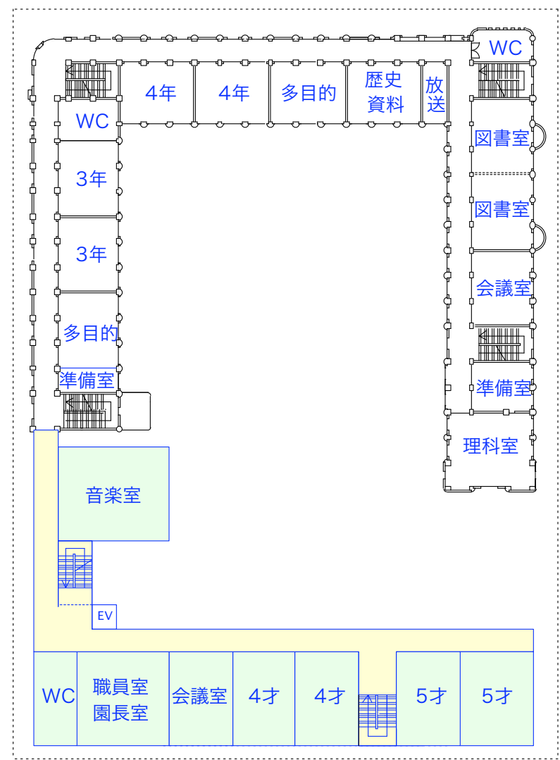
現校舎改修：1,265㎡ 増築：983㎡ 2階平面図
