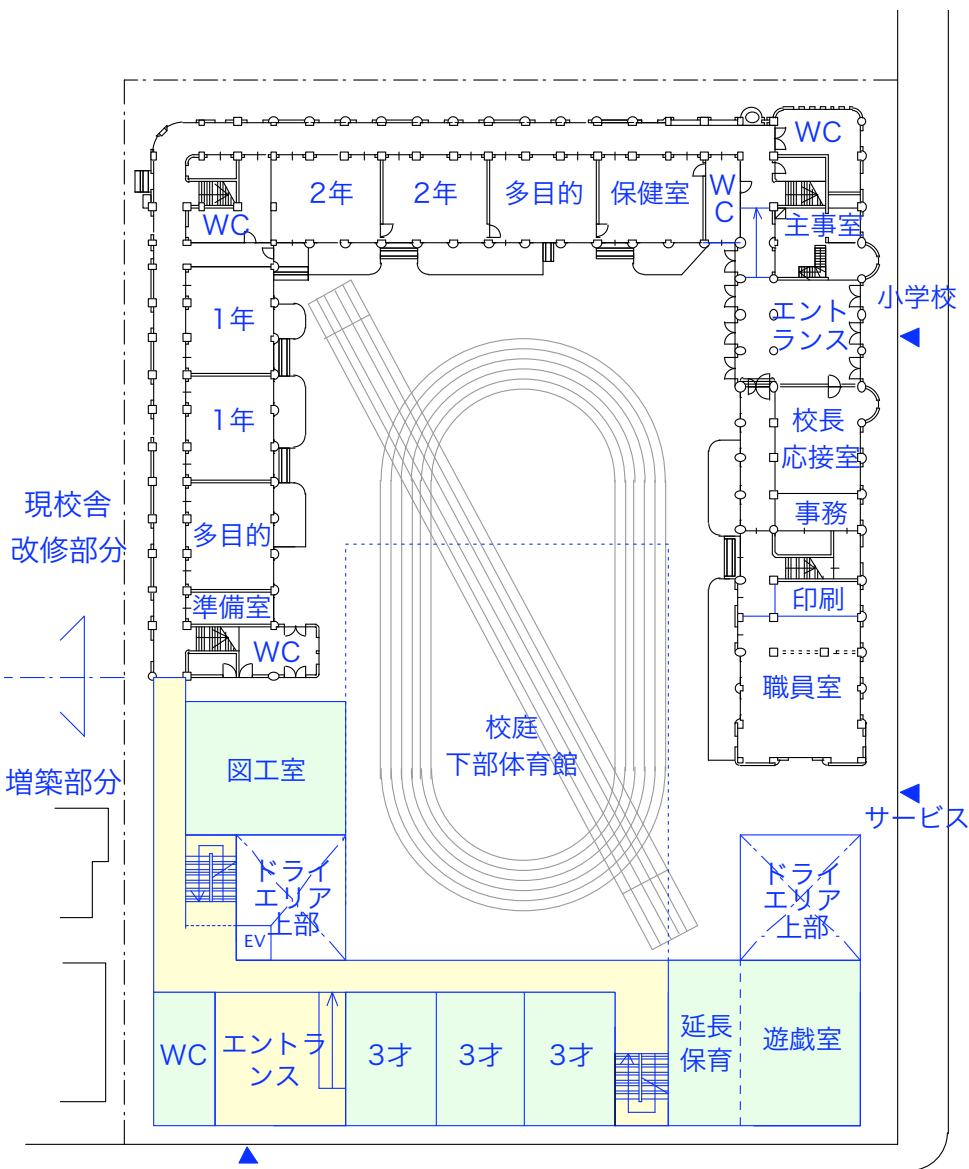
現校舎改修部分 増築部分 幼稚園 現校舎改修：1,285㎡ 増築：983㎡ 1階平面図
