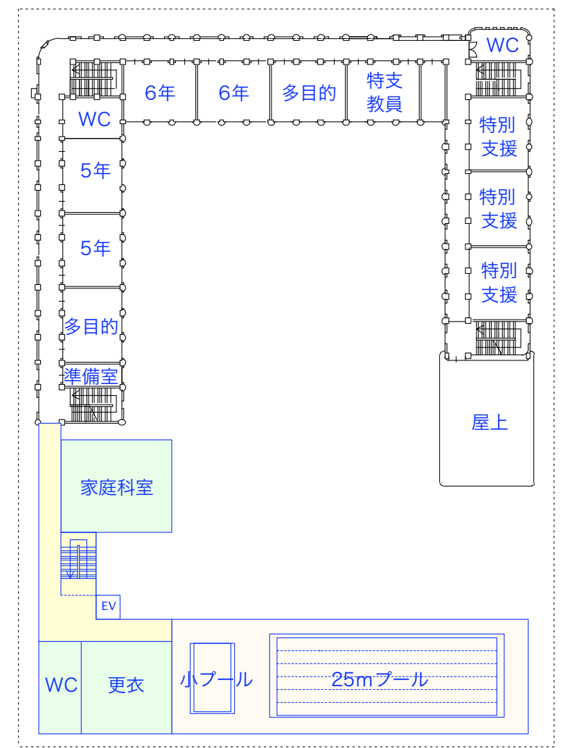
現校舎改修：1,127㎡ 増築：443㎡ 3階平面図
