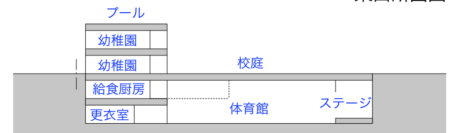
南北断面図
