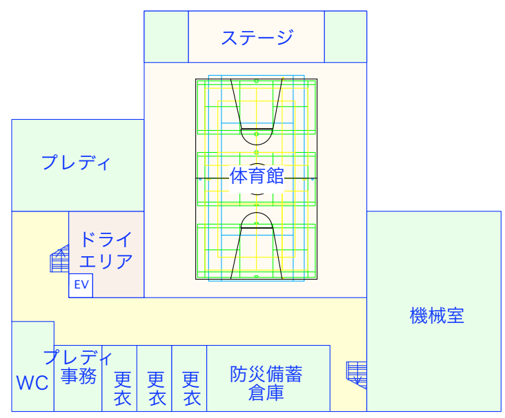
増築：1,975㎡ B2階平面図
